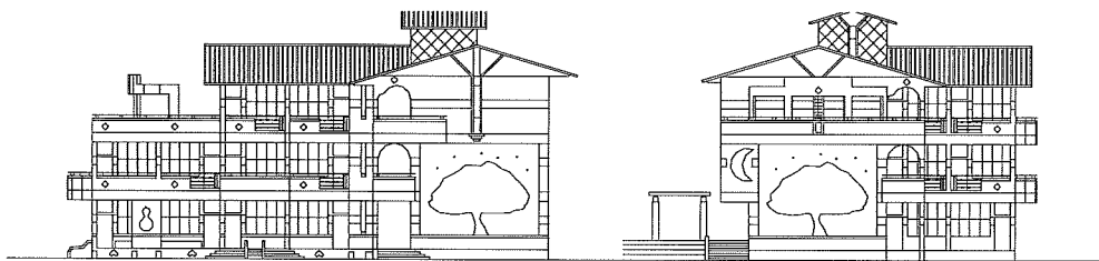
西向立面圖
