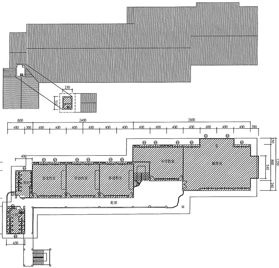
甲棟屋頂面積計算圖
