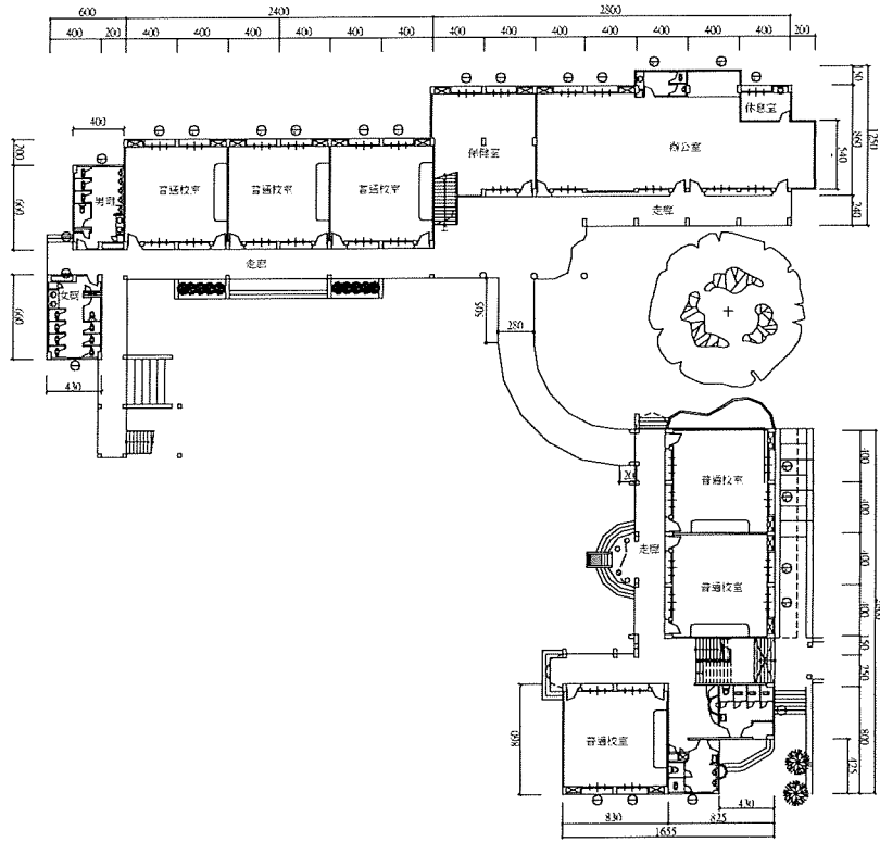
一層平面圖
