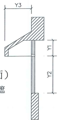
圖 2.4 垂直遮陽修正係數為 (Hw/Hs)^2 之圖示
