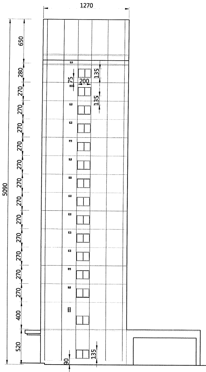
附圖 6 北向立面圖(左圖)
