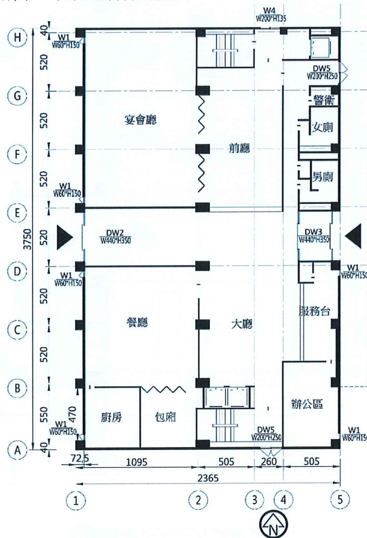
附圖 1 一層平面圖
