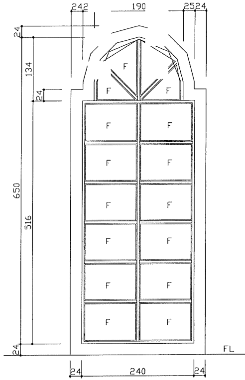
SW 8 240×650 不銹鋼落地門 五金配件齊全 裝配 10mm膠合安全玻璃
