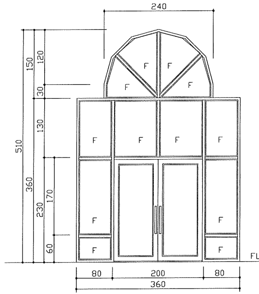
SD0 360×510 不銹鋼落地門 五金配件齊全 裝配 10mm膠合安全玻璃
