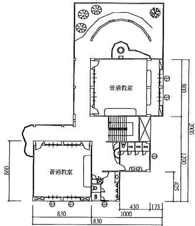
三層平面圖
