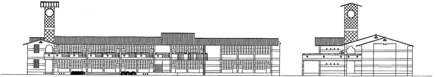
南向立面圖
