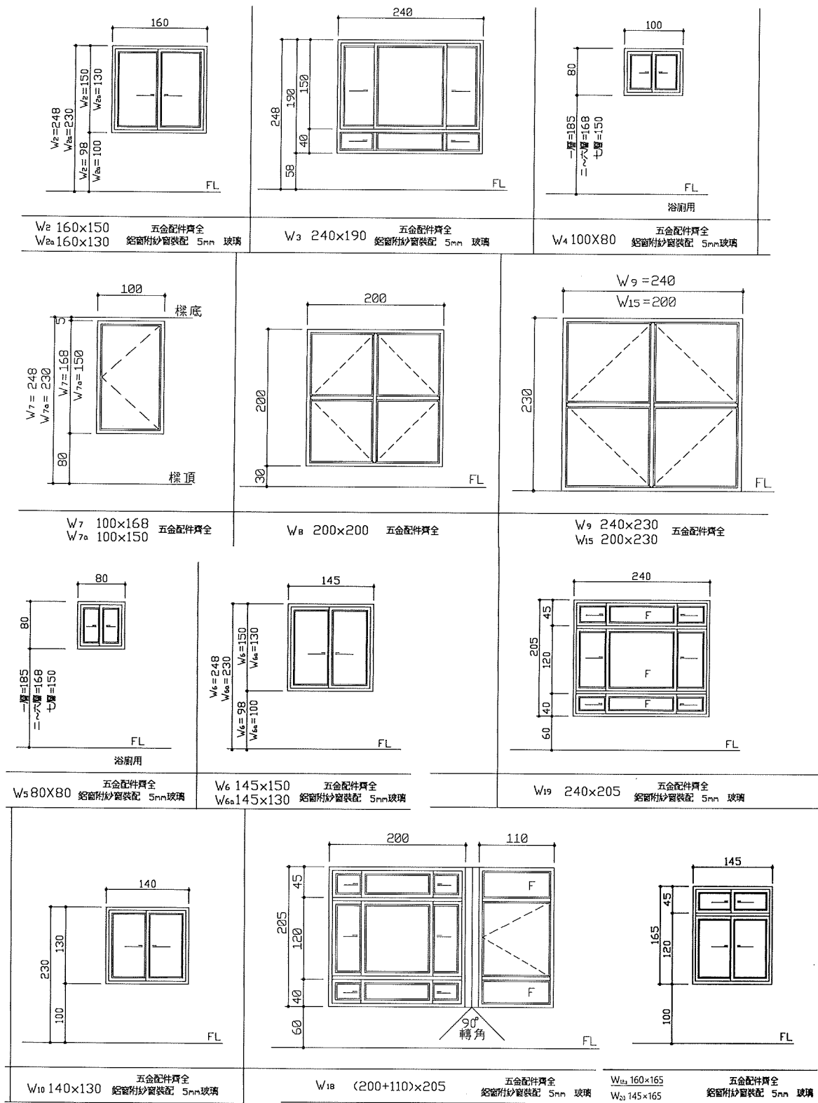
圖 A-9 門窗大樣圖 1
