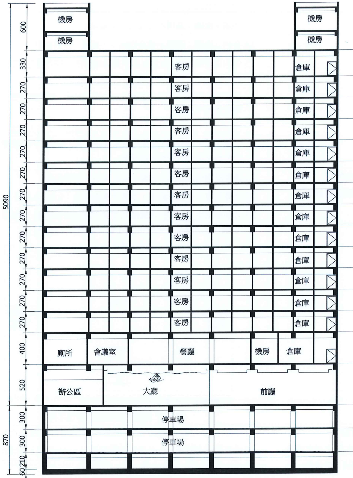
附圖 8 長向剖面圖
