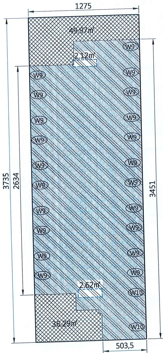
15層內外周區面積圖
