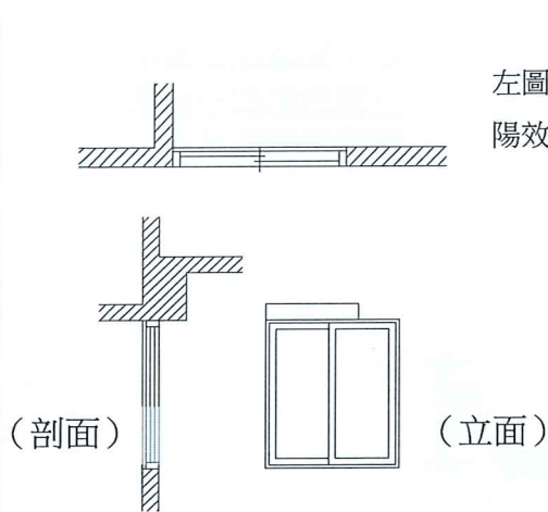
圖 2.5 局部遮陽之 K_{si}' 修正計算
