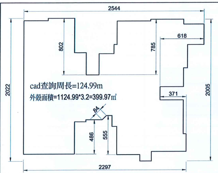
三層外殼面積計算圖
