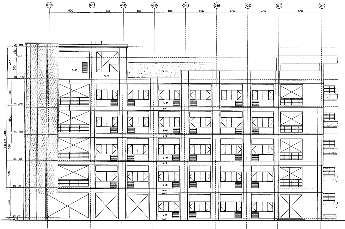
北向立面圖
