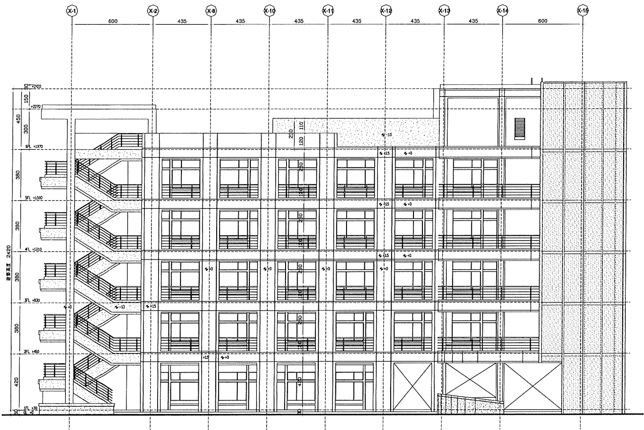
南向立面圖
