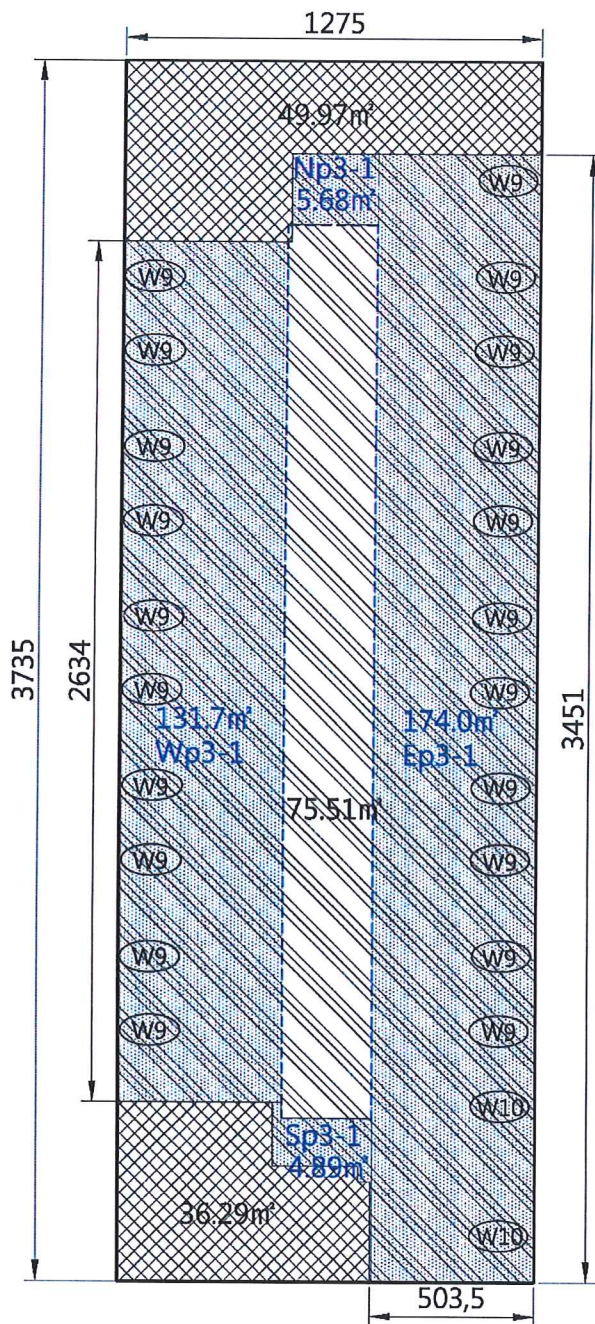
3-14層內外周區面積圖 樓高=2.7m
