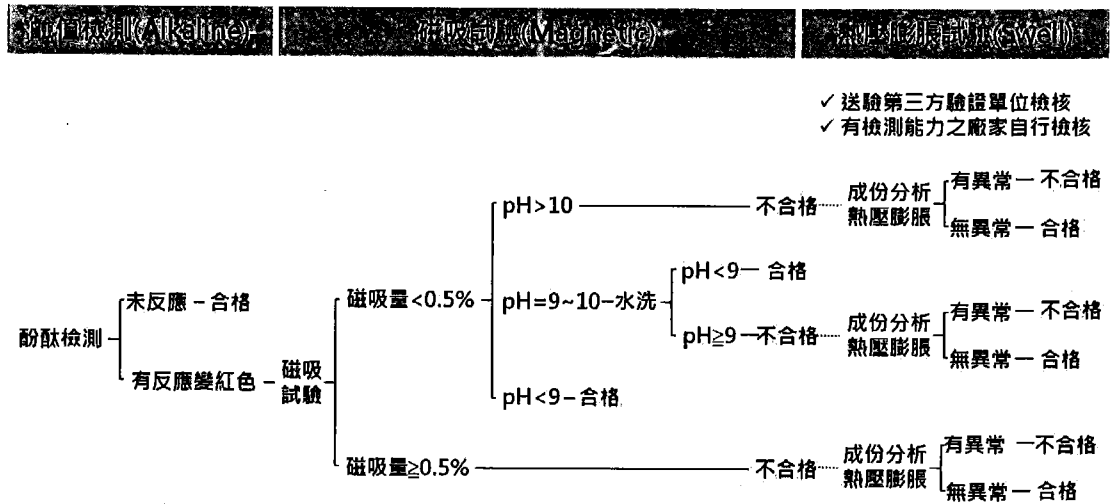
圖 1 AMS 砂石爐渣快篩檢測法流程圖
